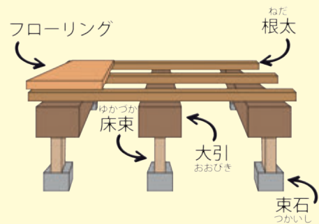
床下の構造
